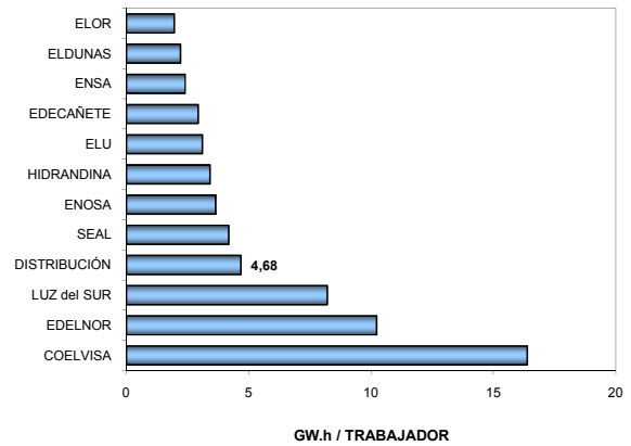
VENTA DE ENERGÍA ELÉCTRICA POR TRABAJADOR EN LAS EMPRESAS POR DISTRIBUCIÓN
